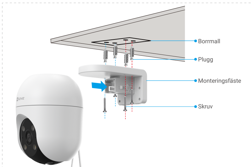
Fig. 1 Takmontering
