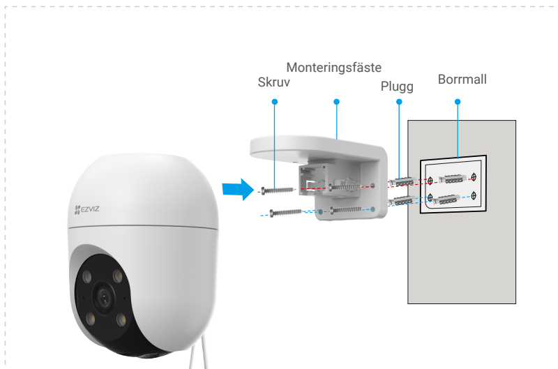
Fig. 2 Vägmontering
